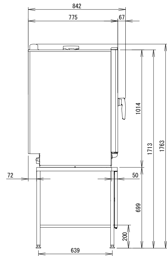
* iCombi Pro / Classic 10-1/1 設置時
